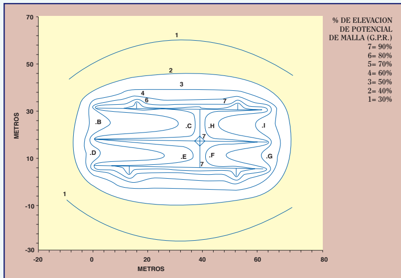
Figura 7-4 Potencial en la superficie del suelo en torno y en el interior de una subestación con diseño antiguo que incorpora barras y electrodos horizontales
