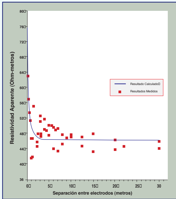
Figura 6-7 Resistividad aparente del suelo graficada en función de la separación de las estacas de prueba. Suelo relativamente uniforme
