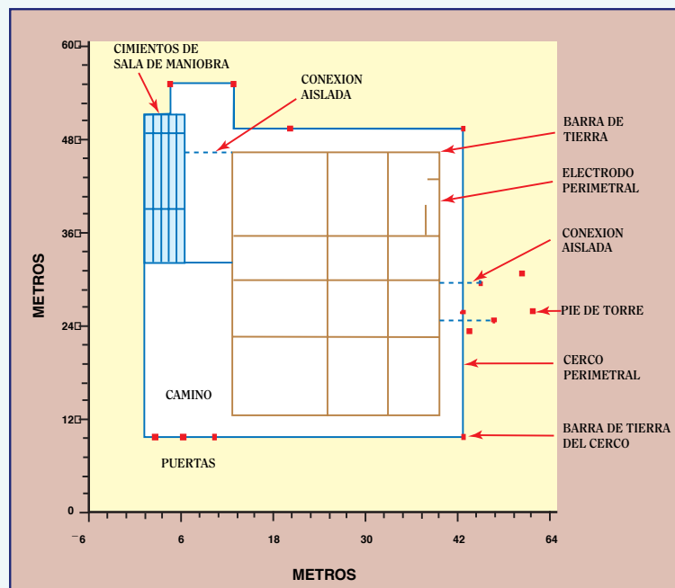
Figura 7-5 Arreglo moderno del tipo malla, para puesta a tierra de subestación
