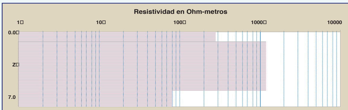
Figura 6-8 Resistividad aparente del suelo graficada en función de la separación de la estacas de prueba. Suelo de tres capas
