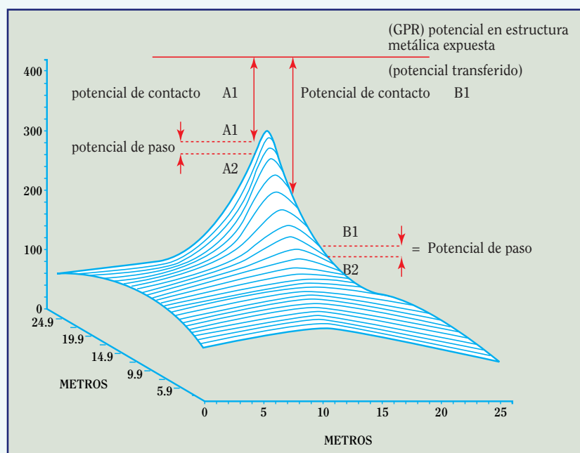
Figura 2-1 Potenciales de Contacto, de Paso y Transferidos en torno a una barra de tierra
