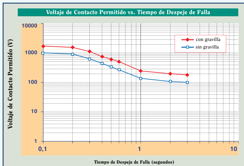
Figura 2-2 Potencial de contacto permitido de acuerdo a EA TS 41-24
