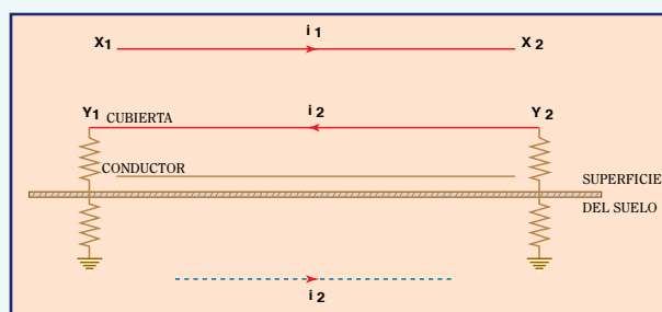
Figura 10-4 Reducción de interferencia inductiva usando una pantalla o blindaje puesto a tierra
