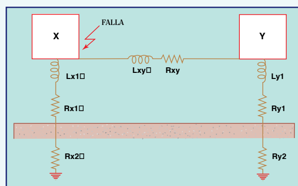
Figura 10-1 Ejemplo para ilustrar la interferencia resistiva
