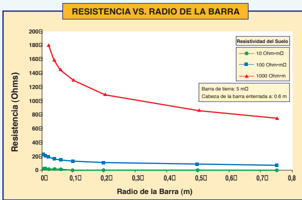
Figura 6-5 Resistencia vs Radio de la Barra
