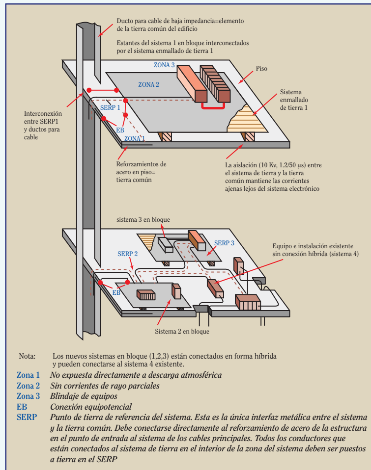
Figura 8-5 Arreglo de sistemas de puesta a tierra híbrido para reducir interferencia (cortesía WJ Furse, basado en trabajo de Eric Montandon)
